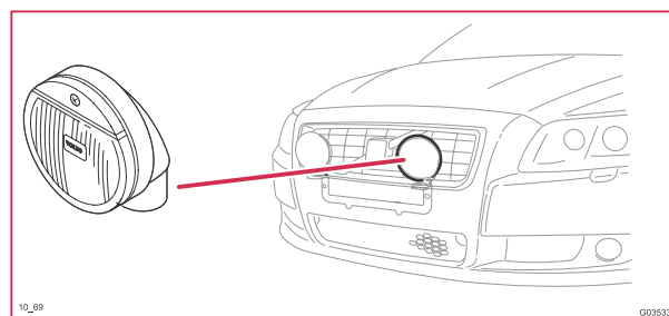
10/69 左前附加燈
